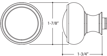
25063 DOOR KNOB SCREEN DOOR
