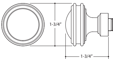
25047 DOOR KNOB SCREEN DOOR
