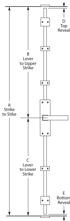
INSWING DOOR
