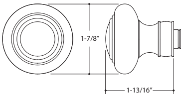
25060 DOOR KNOB SCREEN DOOR
