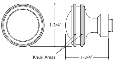
25047-C DOOR KNOB - COIN 25047-D DOOR KNOB - DIAMOND 25047-R DOOR KNOB - ROPE SCREEN DOOR
