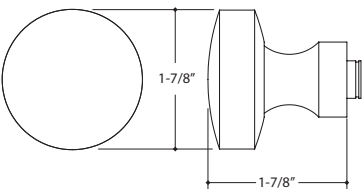
25077 DOOR KNOB SCREEN DOOR
