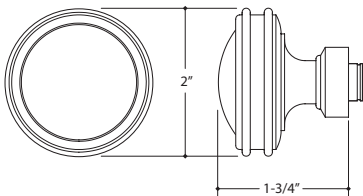
25046 DOOR KNOB SCREEN DOOR
