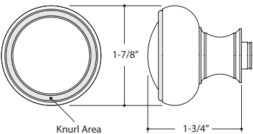
25063-C DOOR KNOB - COIN 25063-D DOOR KNOB - DIAMOND 25063-R DOOR KNOB - ROPE SCREEN DOOR
