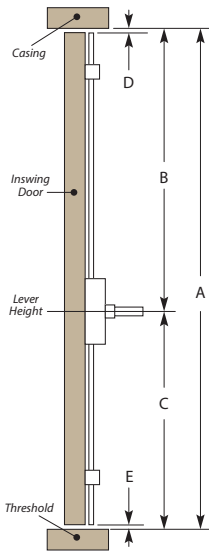
INSWING DOOR
